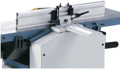
Schwenkbarer Abbrichtanschlag mit stabiler Prismenführung.
