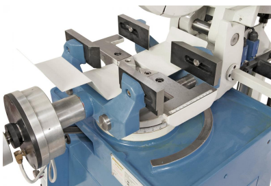
Pneumatischer Schnellspannschraubstock für kurze Rüstzeiten
