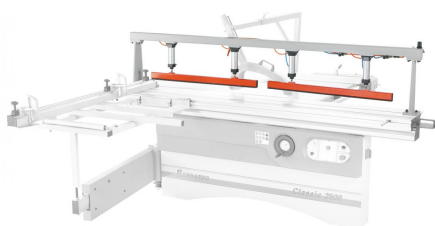
Abbildung mit optional erhältlicher pneumatischer Spannvorrichtung.
