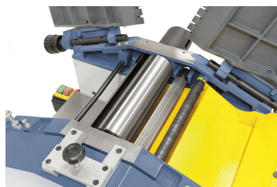
Hobelwerk bestehend aus: 3-Messerwelle, geriffelte Einzugs- und gummierte Auszugswalze.
