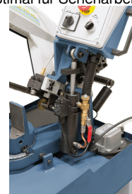
Hydraulikzylinder für stufenloses Absenken des Sägebügels.
