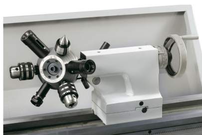
Optional lieferbar: Revolverkopf mit 6 Stationen
