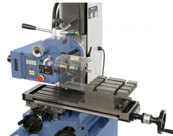
Erhöhter Einsatzbereich durch den schwenkbaren Fräskopf (90° R / 30° L). Der optionale Würfeltisch erleichtert das Fräsen in horizontaler Position.
