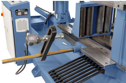
Manuelle Voreinstellung der Materiallänge mittels Mikroschalter, Eingabe und Kontrolle der Stückanzahl am Bedienpult
