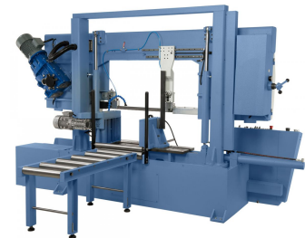
Zum Auflegen von langen Werkstücken ist eine Zufuhrrollenbahn im Lieferumfang enthalten.
