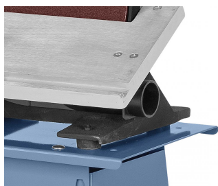
Serienmäßig mit eingebautem Absaugstutzen unter dem bis 45° schwenkbaren Schleiftisch
