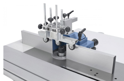
Die Fräuserschutzhaube ist mit eloxierten Aluminium-Anschlagschienen ausgestattet.
