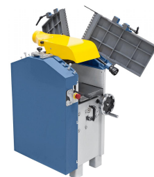
Die hochklappbaren Abrichtische ermöglichen beim Dickenhobeln ein optimales und sicheres Arbeiten, auch bei kurzen Werkstücken.
