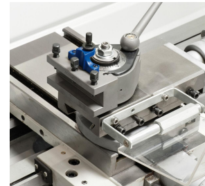
Zum rationellen Arbeiten kann die Maschine mit einem Schnellwechselstahlhalter ausgerüstet werden
