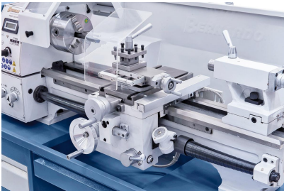
Leichtgängiger Schlitten mit Obersupport und Vierfachstahlhalter, Handräder mit einstellbarer metrischer Feinskalierung
