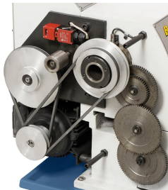
Einfaches Einstellen der Drehzahlstufe mittels Keilriemen
