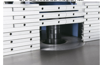
Die Integral-Sicherheitsschienen aus eloxiertem Aluminium lassen sich individuell an jede Fräserform anpassen und gewährleisten
