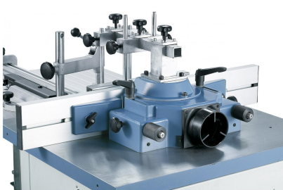
Die Fräferschutzhaube ist mit einer Feineinstellung ausgestattet. Die Späneabfuhr erfolgt über den integrierten Absauganschluss.
