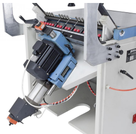
Pneumatisches Schwenken der Bohreinheit von 0° - 45° - 90°
