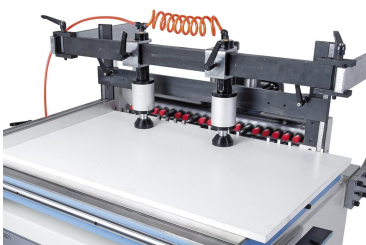
Pneumatische Spanner verschiebbar zum Bohren auch von kleineren Werkstücken
