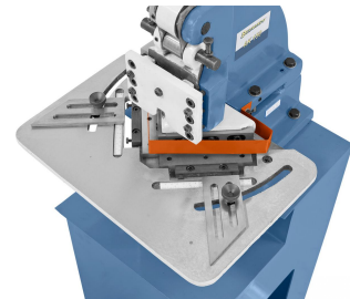
Einstellbare Anschläge mit Skalen
