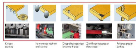
Kleben gleitend Kantenendschnitt end cutting Doppelflächaggregat finishing R side Ziehlingaggregat flap scraper Rollenaggregat buffing
